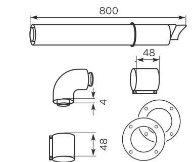
Vodorovné odkouření stěnou/střechou
