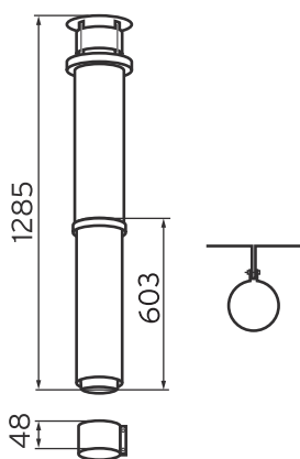
Svislé odkouření včetně střešního nástavce
