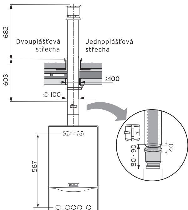
Montáž kotle a průchodu plochou střechou
